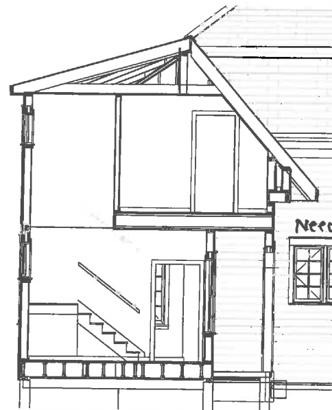
Section @ Conntector
